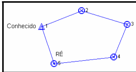
Figura 5.11 – Exemplo de Poligonal Fechada.
