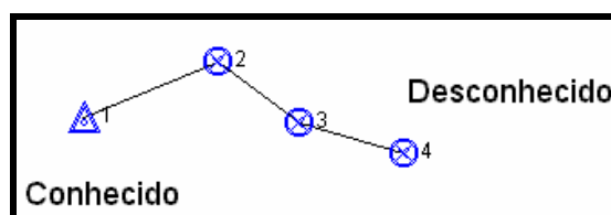
Figura 5.10 – Exemplo de Poligonal Aberta sem Controle.
