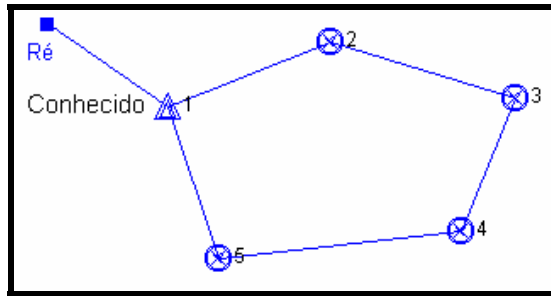
Figura 5.13 – Exemplo de Poligonal Fechada (Com Ponto de Apoio)
